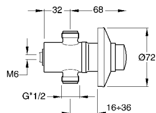
QK15051 Samouzavírací podmínkový sprchový ventil 1 690,- / 73 € QK11051 Samouzavírací podmínkový pisoárový ventil 1 640,- / 72 €
