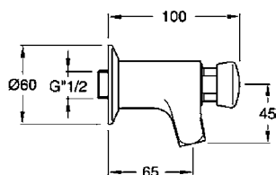
QK23551 Samouzavírací nástěnný ventil na umyvadlo 1 190,- / 53 €
