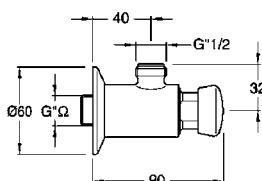
QK16051 Samouzavírací sprchový ventil 1 120,- / 49 € QK10051 Samouzavírací pisoárový ventil 1 060,- / 46 €
