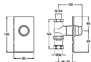
QK82051 Samouzavírací podmínkový WC ventil 2 990,- / 130 €
