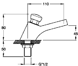
QK23051 Samouzavírací stojánkový ventil na umyvadlo 1 390,- / 60 €
