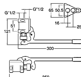
QK40051 Ventil s pedálem pro nástěnnou nebo podlahovou instalaci 2 590,- / 113 €
