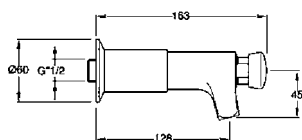
QK24051 Samouzavírací prodloužený nástěnný ventil na umyvadlo 1 640,- / 73 €
